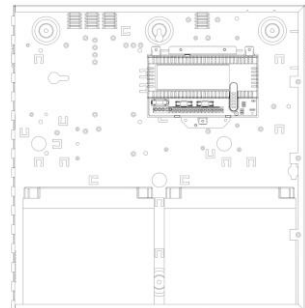
STV2405 dans un boîtier E avec batteries 17 Ah
